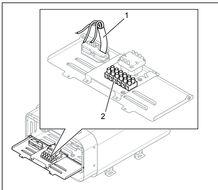
Afbeelding 6: De printplaat
