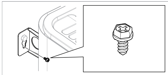
Afbeelding 11: Sluitbouten van de beugels
