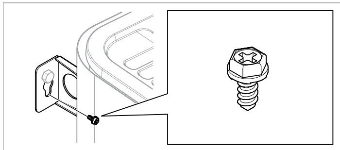
Rysunek 11: Śruba zabezpieczająca wspornika
