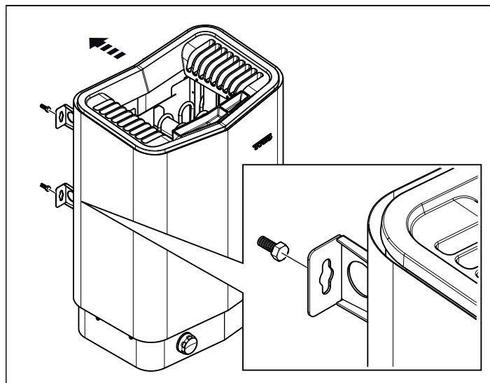
Afbeelding 10: De kachel ophangen
