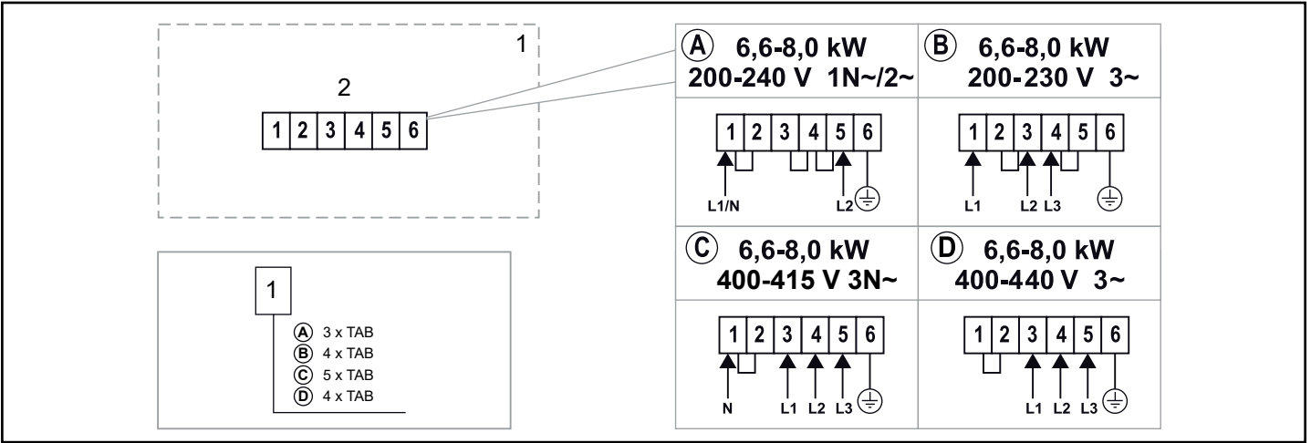
Rysunek 12: Schemat elektryczny 1. Piec 2. Zacisk do podłączenia kabla elektrycznego
