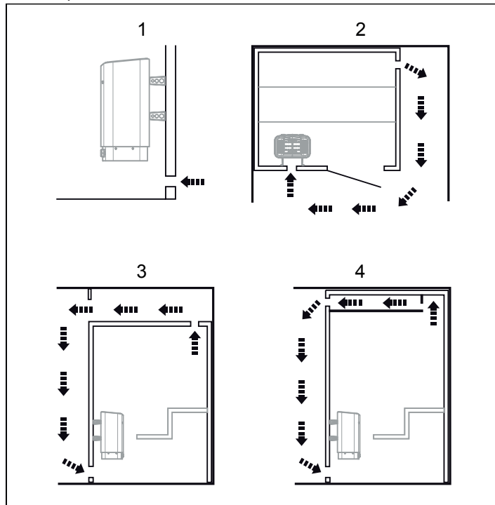
Fig 4: Emplacement des bouches d'entrée et de sortie d'air
