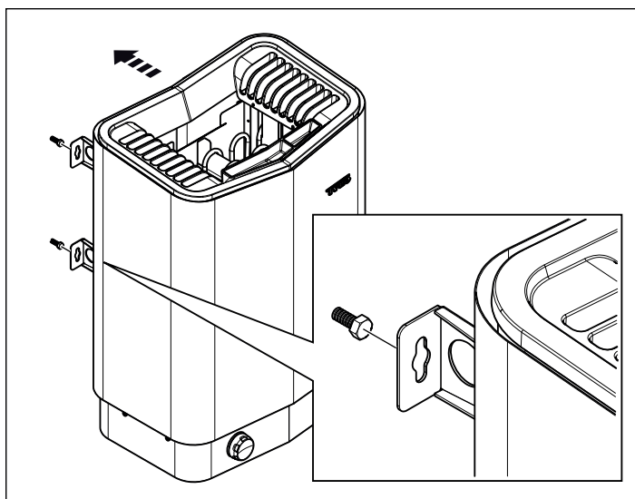
Rysunek 10: Zawieszanie pieca
