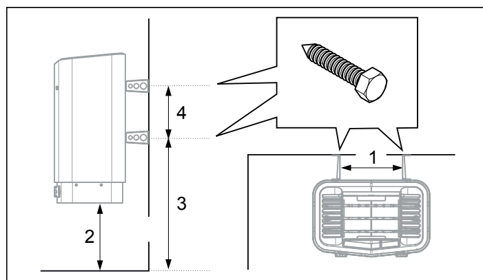
Afbeelding 8: Aangegeven maten
