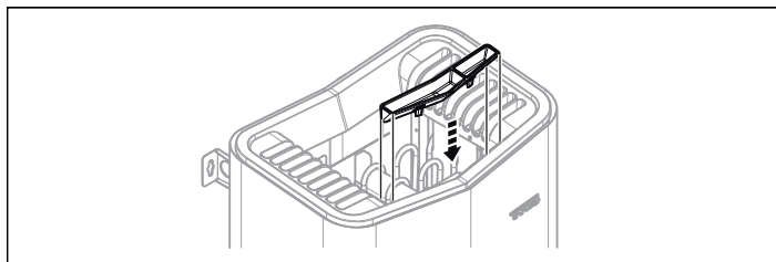
Rysunek 9: Montaż zbiornika na olejki / nawilżacza powietrza
